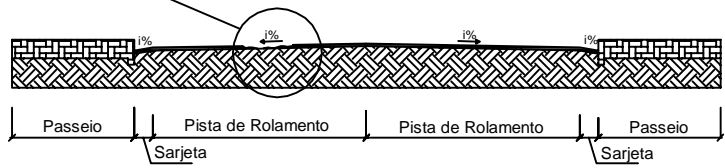
Seção Transversal Tipo Via Urbana
