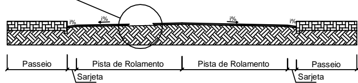
Seção Transversal Tipo Detalhe Remendo
