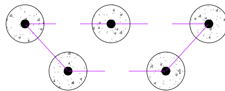
ESQUEMA FUNDAÇÕES MICRO ESTACAS Ø30CM ARMADAS AS MEDIDAS ENTRE EIXOS DEVERÃO SER CONFERIDAS DE ACORDO COM O FABRICANTE
