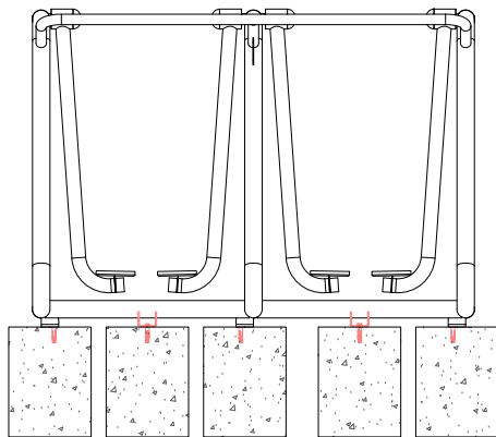
VISTA FRONTAL E LATERAL - SIMULADOR DE CAMINHADA DUPLO
