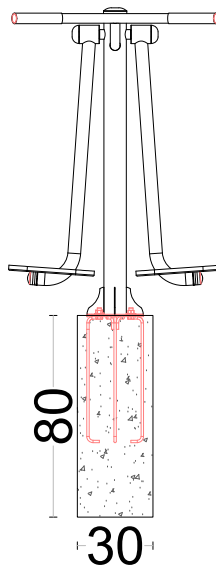
VISTA FRONTAL - SURF DUPLO
