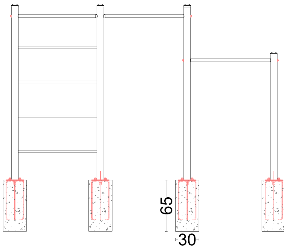
VISTA FRONTAL - FUNDAÇÃO BARRA MODULAR
