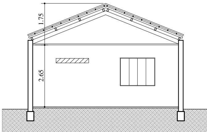
CORTE B-B
