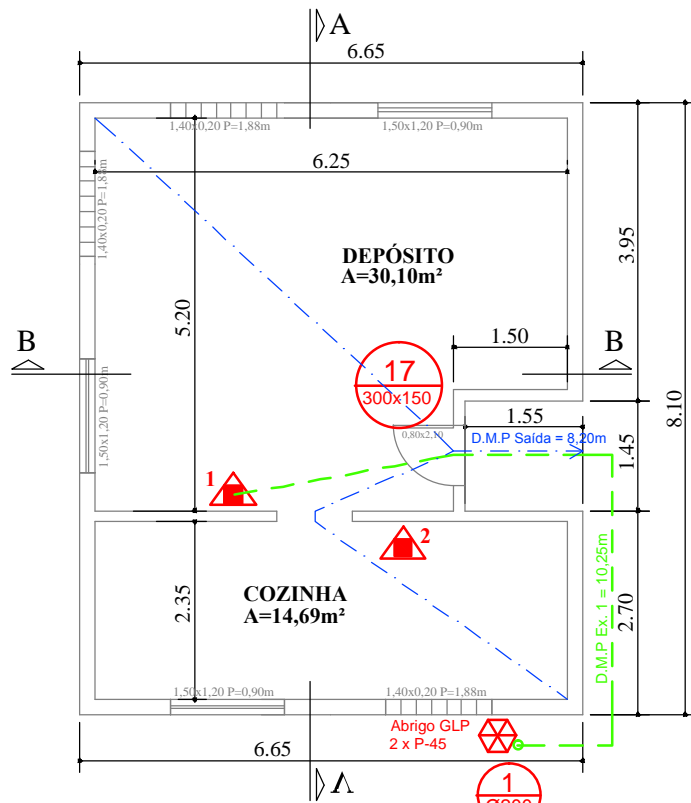
PLANTA BAIXA - PPCI
